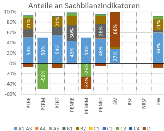
Abb. 6-3: Sachbilanzindikatoren anteilig je Modul
