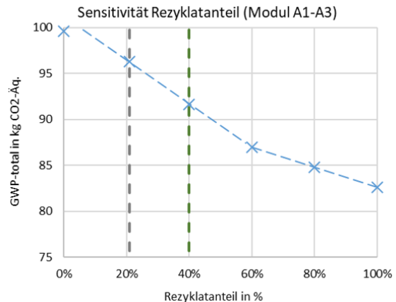
Abb. 6-1: GWP-total der Fensterherstellung Modul (A1–A3) in Abhängigkeit vom Rezyklatanteil
