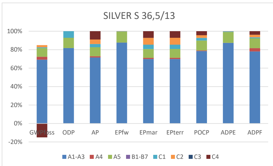
Abbildung 3: Beitrag der Lebenszyklusphasen zum Gesamtergebnis, SILVER S 36,5/13
