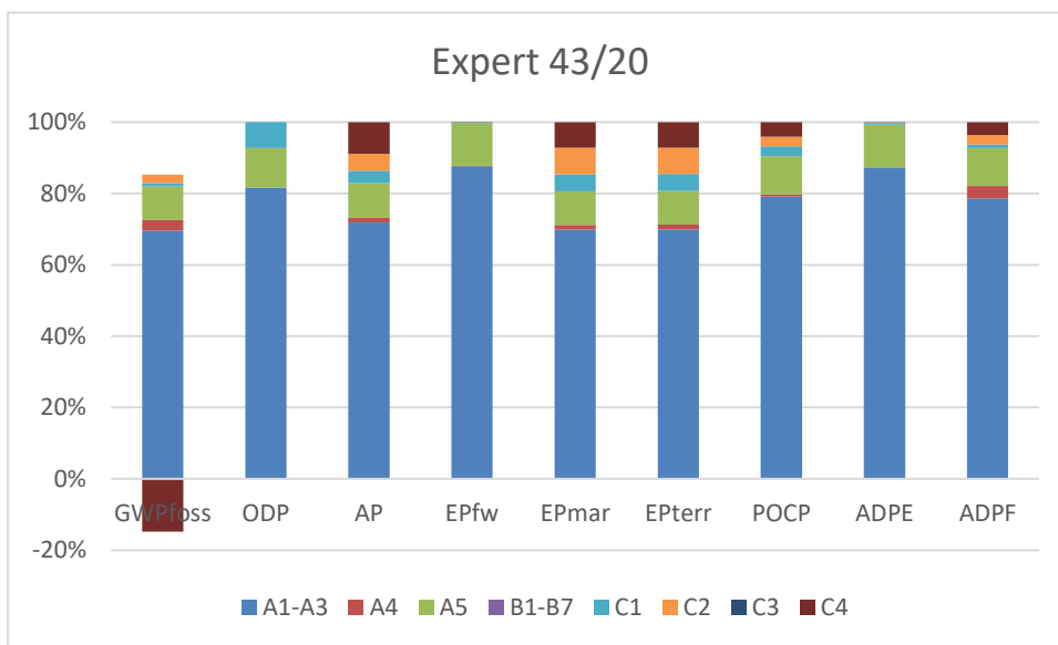
Abbildung 4: Beitrag der Lebenszyklusphasen zum Gesamtergebnis, Expert 43/23
